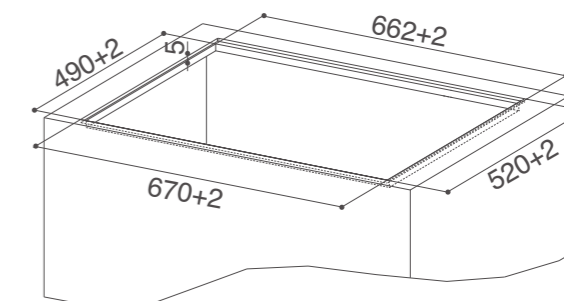
HOO-B GLASS + 2 PIANI INDUZIONE FABER FBH32 INSTALLAZIONE FILOTOP
