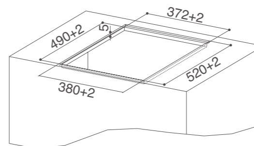
HOO-B GLASS + 1 PIANO INDUZIONE FABER FBH32 INSTALLAZIONE FILOTOP
