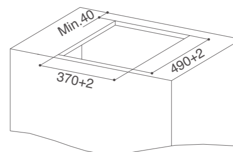
HOO-B + 1 PIANO INDUZIONE FABER FBH32
