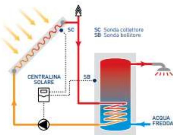
Schema d'impianto a circolazione forzata
