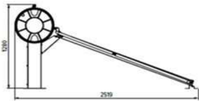
150 E 200 LITRI 1 COLLETTORE
