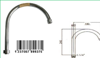
Canna Alta A Tubo Per Lavabo Da Mm Da 230X190 Mm Girevole
