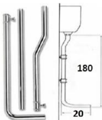
Tubo Esterno Cromo Diba
