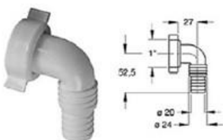
Curva Abs X Lavatrice Bianco 1" Fx22 Vedi Articolo Rplbh
