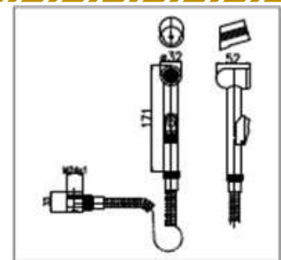
Raccordo universale girevole M.24x1 completo di flessibile 1/2"x1/2" 150 cm, doccia a pulsante e supporto
