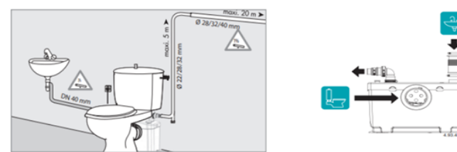
VASO+ATTACCO LAVABO
