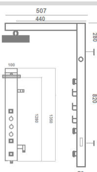
Colonna doccia con testa girevole Il kit include: Colonna doccia sagomata con testa girevole; soffione anticalcare 200 mm.; doccia 3 getti anticalcare 110; deviatore;
