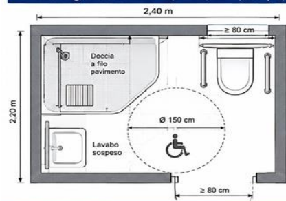
Pianta bagno accessibile – 2,20 x 2,40 m (esempio)
